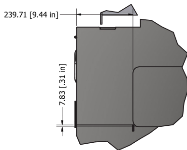
DETAIL BD SCALE 0.13 : 1
